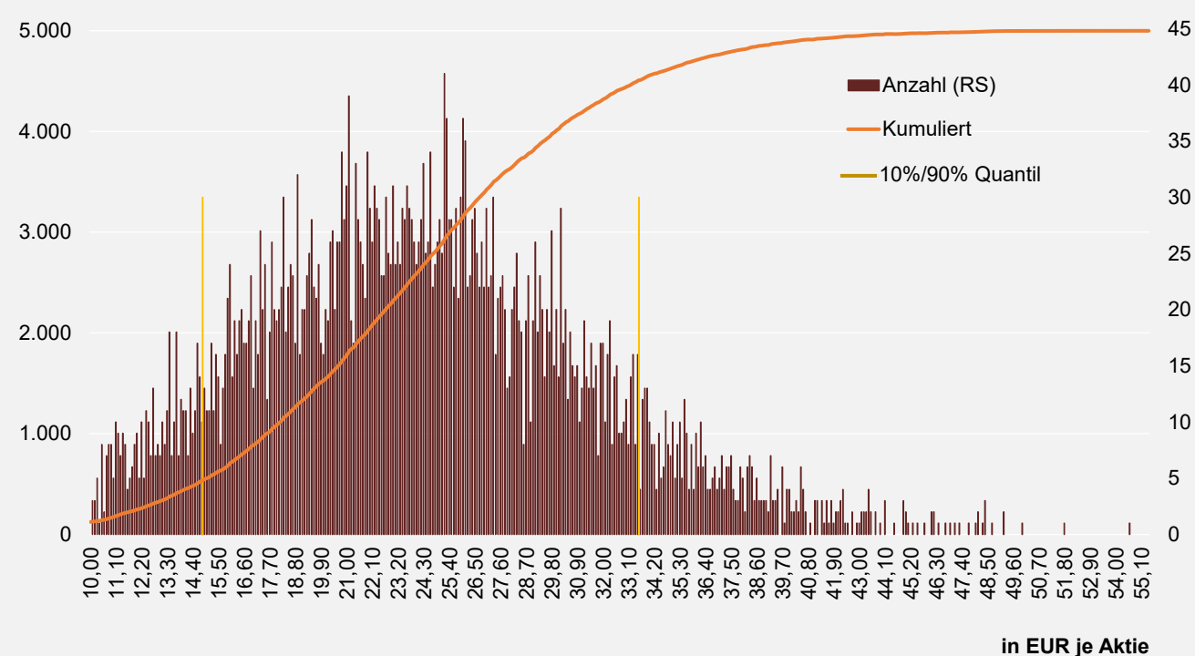
ABBILDUNG 3: MONTE-CARLO-SIMULATION (5.000 SIMULATIONEN)
