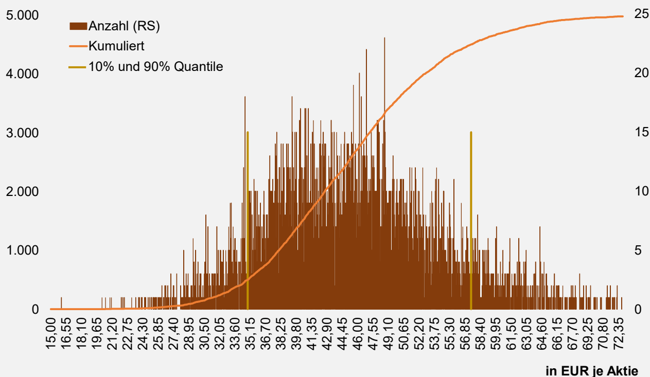
ABBILDUNG 1: MONTE-CARLO-SIMULATION (5.000 SIMULATIONEN)
