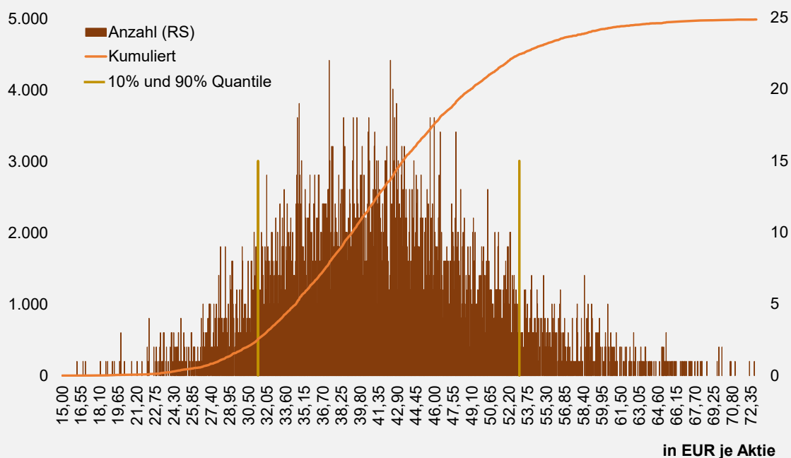
ABBILDUNG 3: MONTE-CARLO-SIMULATION (5.000 SIMULATIONEN)
