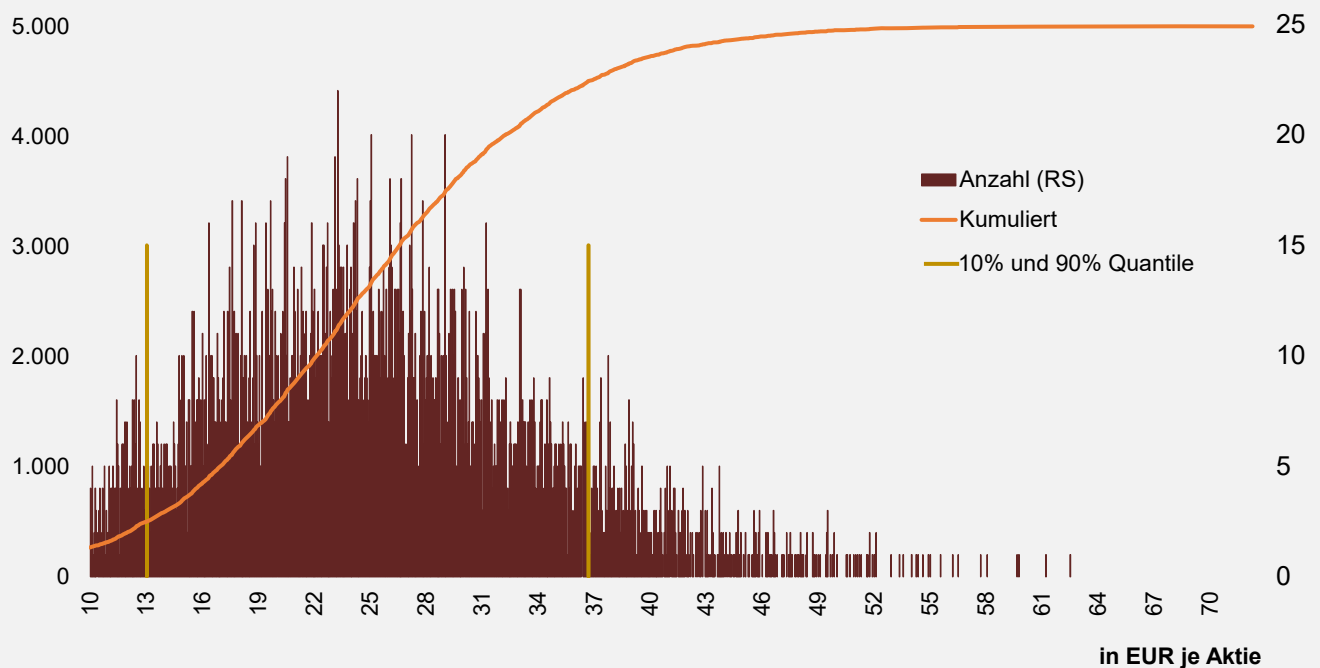
ABBILDUNG 1: MONTE-CARLO-SIMULATION (5.000 SIMULATIONEN)
