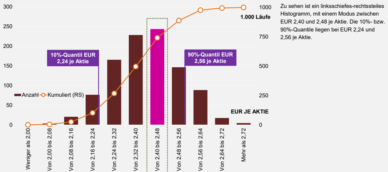
ABBILDUNG 1: MONTE-CARLO-SIMULATION
