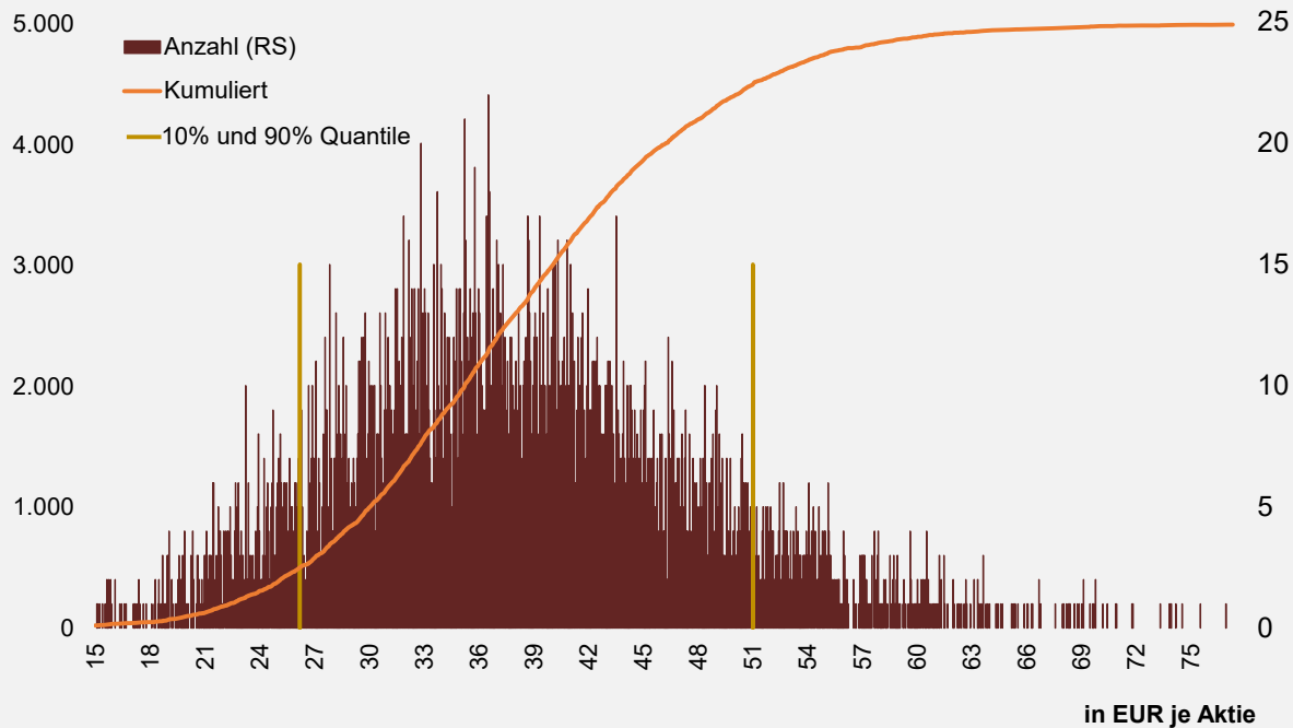
ABBILDUNG 1: MONTE-CARLO-SIMULATION (5.000 SIMULATIONEN)
